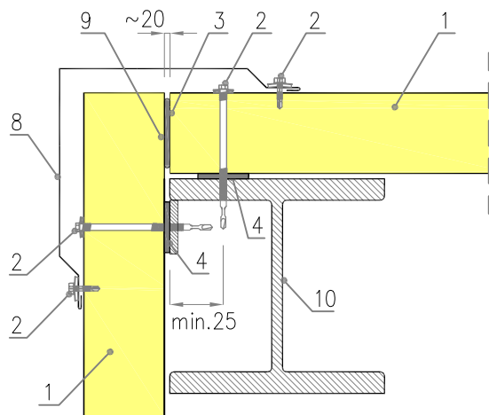
Wariant II – poziomy układ płyt:
