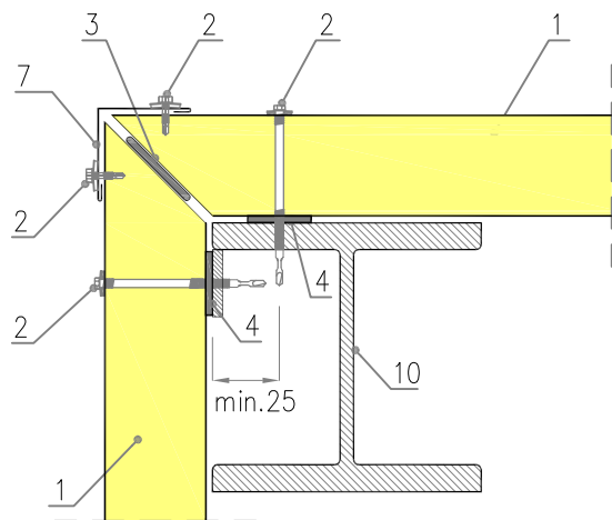
Wariant I – poziomy układ płyt:
